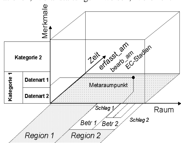
Abbildung 1: Zuordnung von Metadaten im Begriffsraum
